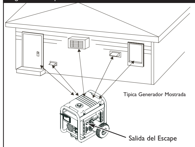
Figura 11 — Espacio Libre Alrededor del Generador
